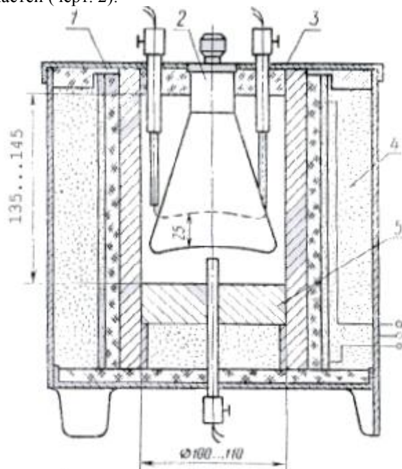
1 -огнеупорный цилиндр; 2 -колба; 3 -крышка; 4 -металлический цилиндр; 5 - вставка
